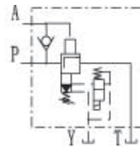
DAW...-50B/...Y...
