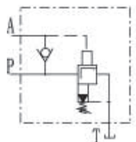
DA...-50B/...
