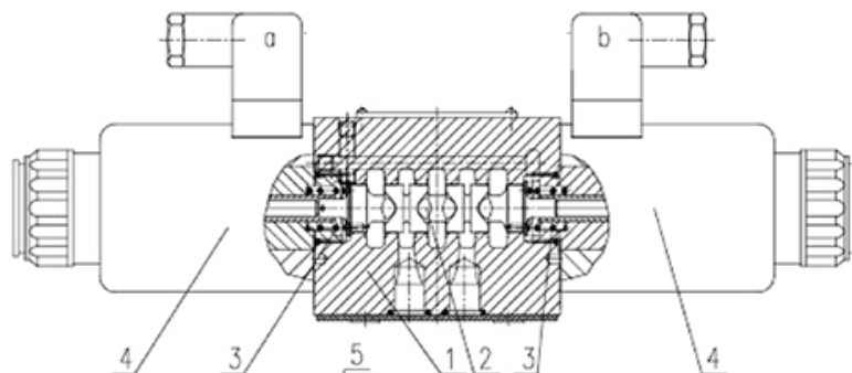
HD-4WRA...-2X/G24K4
